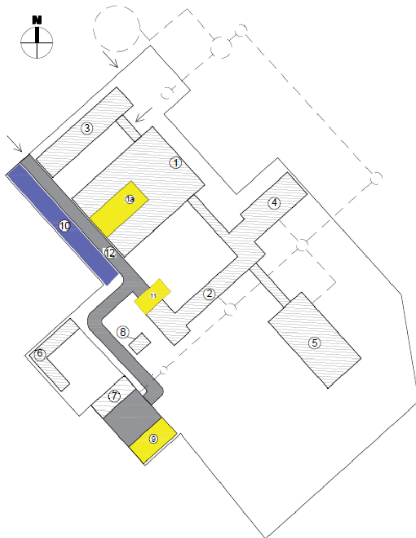
ЗУРАГ 1. ЕРӨНХИЙ ТӨЛӨВЛӨГӨӨ /масштабгүй/
